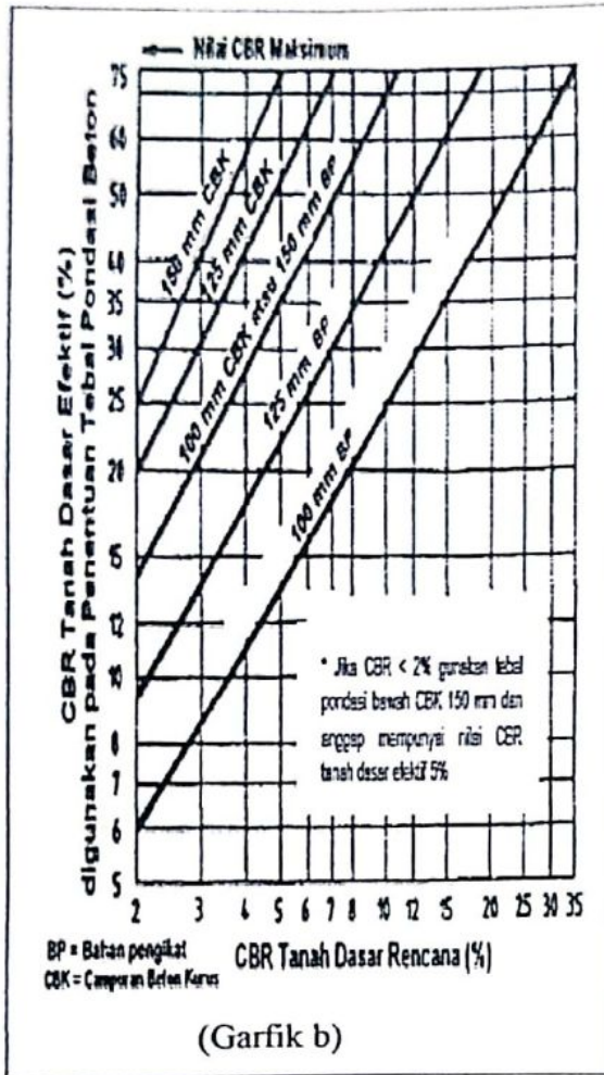
Gambar 3. Grafik-grafik untuk Perhitungan Tebal Perkerasan Kaku
