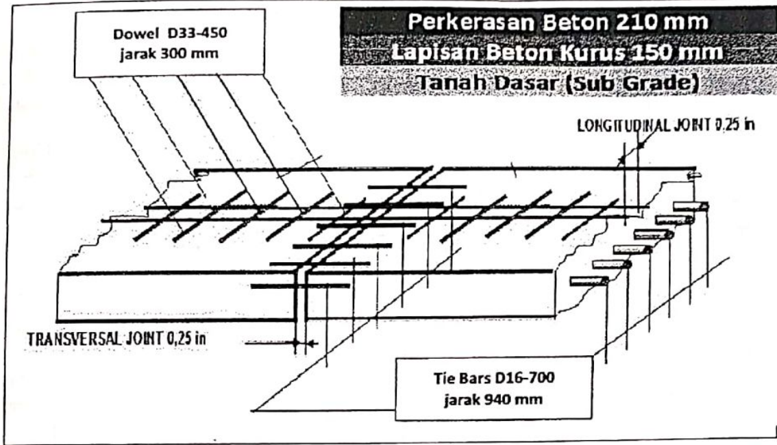
Gambar 5. Hasil Perencanaan Beton Bersambung Tanpa Tulangan
