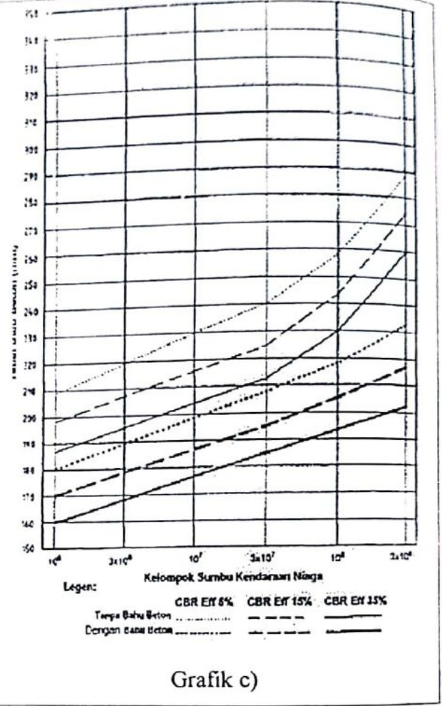
Gambar 3. Grafik-grafik untuk Perhitungan Tebal Perkerasan Kaku
