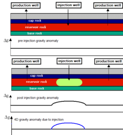
Gambar 1: Model dan respon gravitasi 4D akibat injeksi fluida pada reservoir dengan rapat massa fluida injeksi lebih besar dari rapat massa fluida pengisi pori sebelumnya yaitu minyak dan air
