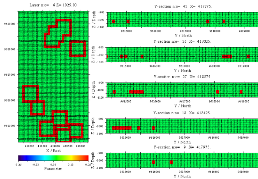
Gambar 4: Model awal inversi akibat injeksi periode Mei hingga September tampak dari atas dan tampak dari samping
