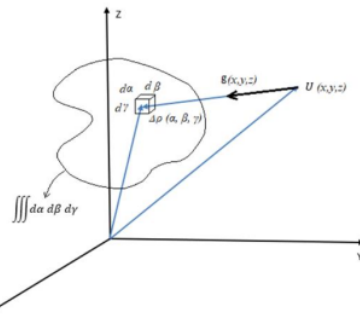
Gambar 2: Gravitasi di titik P(x,y,z) akibat elemen massa \rho(\alpha,\beta,\gamma)
