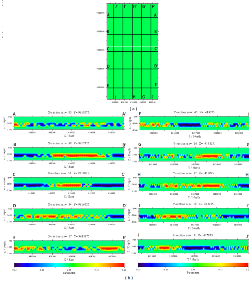
Gambar 5: Hasil inversi pada periode Januari hingga Mei dalam 10 sayatan
