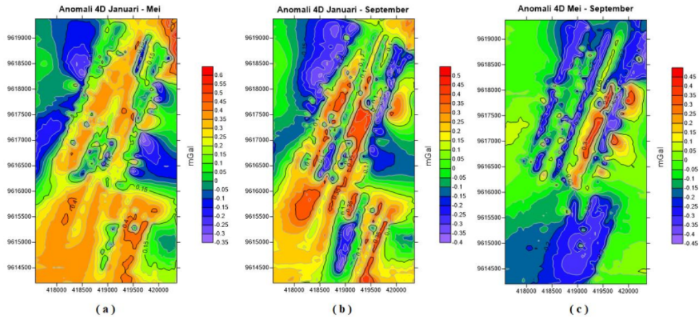
Gambar 3: Anomali Gravitasi 4D pada periode (a) Januari hingga Mei (b) Januari hingga September (c) Mei hingga September
