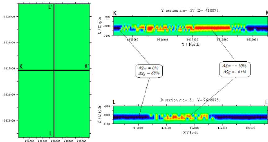
Gambar 6: Interpretasi pengurangan saturasi minyak dan saturasi gas model reservoir hasil inversi periode Januari hingga Mei
