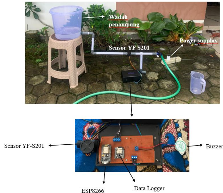
Gambar 4 .Rancangan monitoring penggunaan air dan tagihan PDAM
