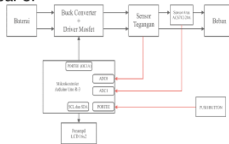
Gambar 5. Blok diagram perencanaan perancangan buck converter.
