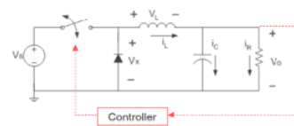
Gambar 2. Topologi rangkaian buck converter (Taufik, 2008).
