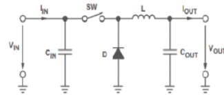
Gambar 6. Rangkaian buck converter
