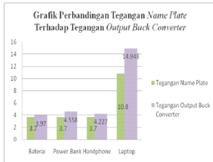
Gambar 11. Grafik perbandingan tegangan name plate terhadap tegangan output buck converter
