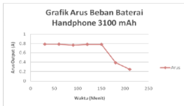
Gambar 9. Grafik arus pengisian menggunakan beban Handphone
