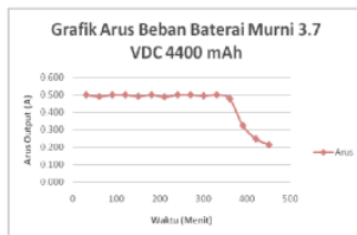
Gambar 7. Grafik arus pengisian baterai murni 3.7 Volt DC
