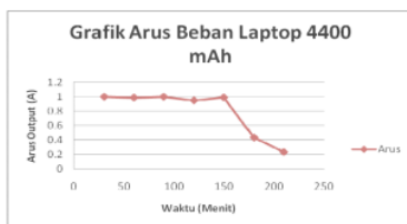
Gambar 10. Grafik arus pengisian menggunakan beban Laptop
