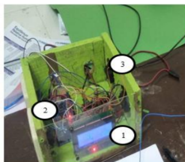
Gambar 2. Rangkaian sistem kendali
