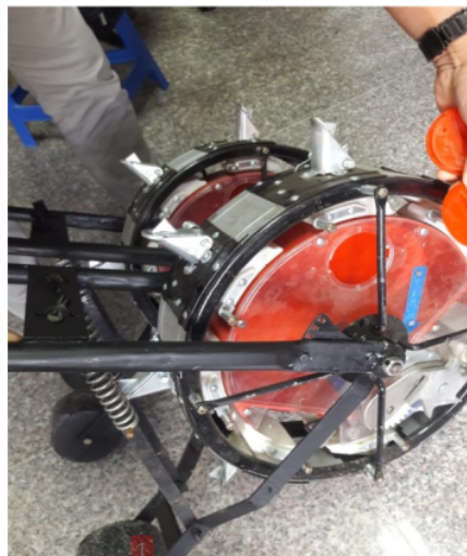
Gambar 3. Uji kinerja alat tanam biji jagung sistem dorong baris ganda di laboratorium
