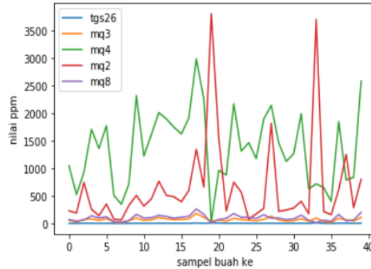
Gbr. 5 Grafik Konversi Nilai Adc Terukur Menjadi Ppm Setiap Sampel Buah Pada Pengukuran Hari ke-7
