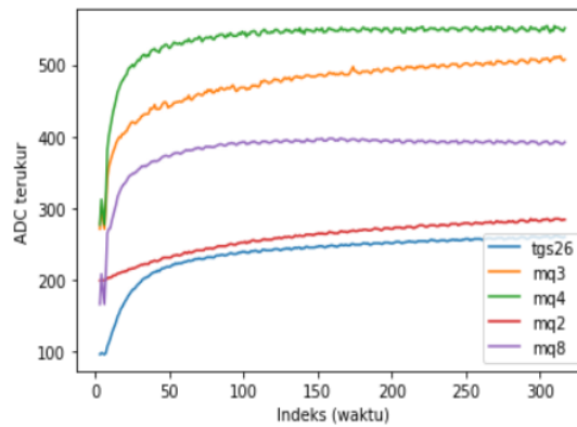
Gbr. 3 Grafik Pengukuran Adc Terukur Hasil Pembersihan
