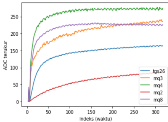
Gbr. 4 Grafik Normalisasi Nilai ADC Terukur
