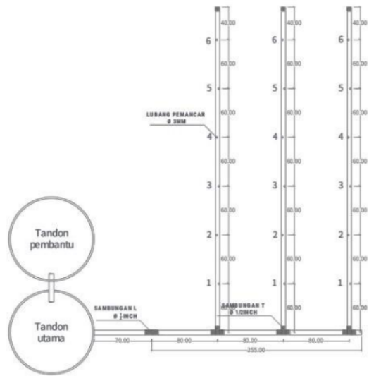
Gambar 1 Sketsa jaringan irigasi perforasi tampak atas
