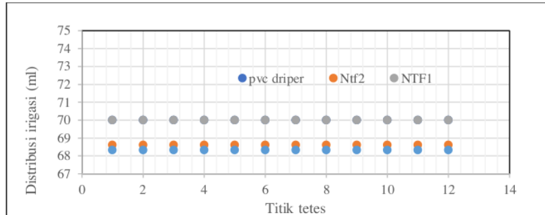
Gambar 5. Distribusi irigasi tetes NTF dan Pvc
