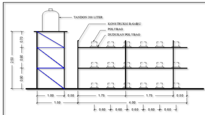
Gambar 3. Skema aringan irigasi tetes bertingkat.
