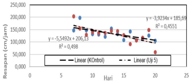
Gambar 5. Perbandingan Regresi Uji 5 Terhadap Kontrol
