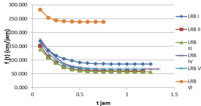
Gambar 1. Grafik Horton hasil pengujian
