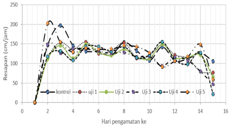
Gambar 2. Pola Resapan dari Biopori Terhadap Kontrol
