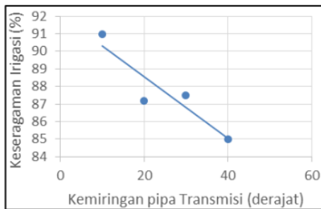
Gambar 7. Hubungan Kemiringan Pipa Transmisi dan Keseragaman Irigasi
