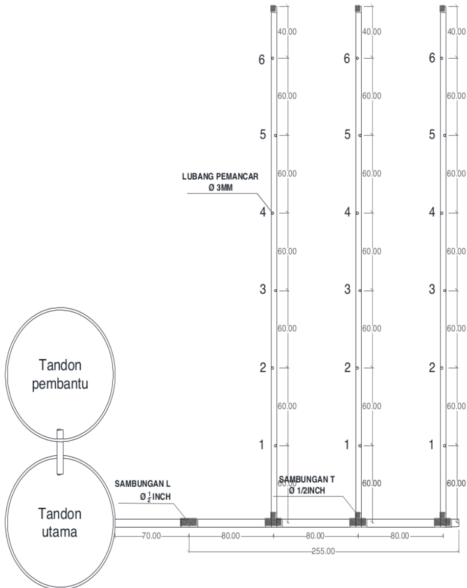
Gambar 2. Denah Jaringan Irigasi Perforasi
