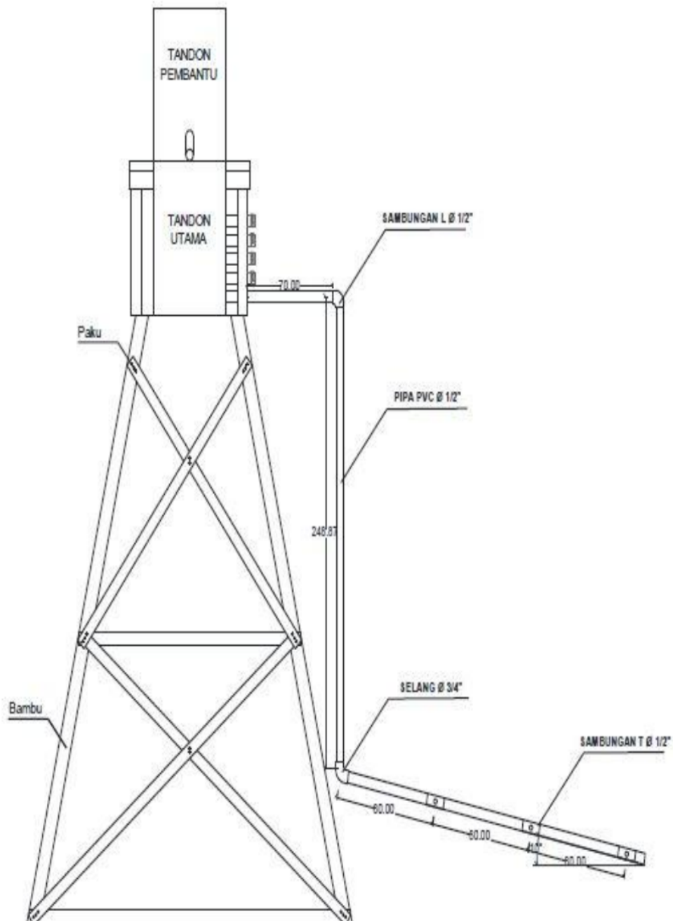
Gambar 3. Rancangan Uji Jaringan Irigasi Perforasi Tampak Samping
