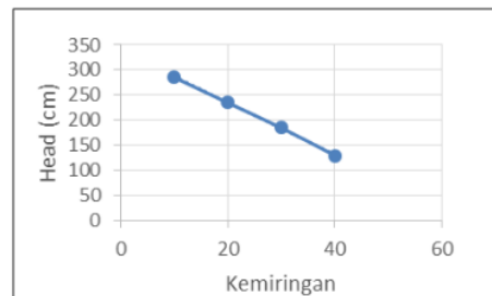
Gambar 5. Hubungan Kemiringan dengan Tinggi Head
