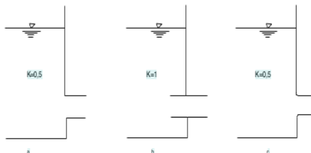
Gambar 1. Bentuk bentuk lubang pemasukan pipa
