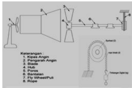
Gambar 6. Set-Up Alat Uji dan Benda Uji
