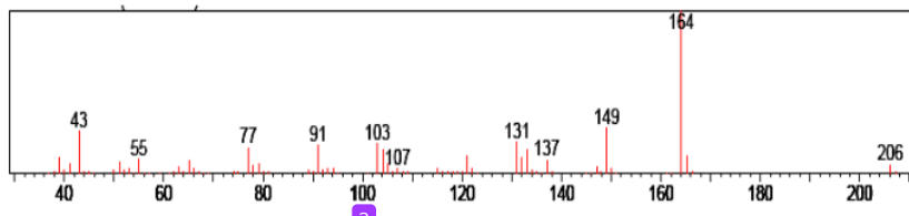
Gambar 4. Spektrum massa eugenil asetat
