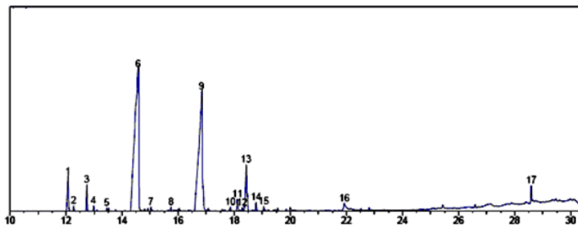
Gambar 3. Kromatogram produk nitratasi eugenol
