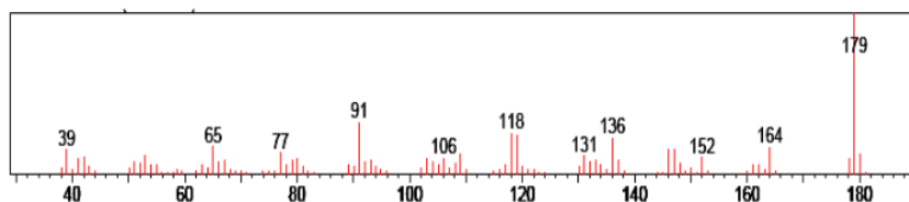
Gambar 6. Spektrum massa 4-allyl-2-metoksi-6-aminofenol (3).
