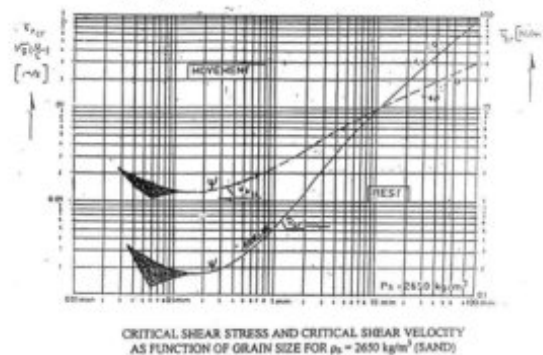
Gambar 11. Grafik Shields untuk Kontrol Stabilitas Butiran pada Penampang IPias Kanan Sungai Belanting
