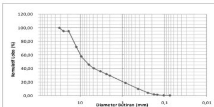
Gambar 8. Kurva Distribusi Kumulatif pada Pias 2 Survei II
