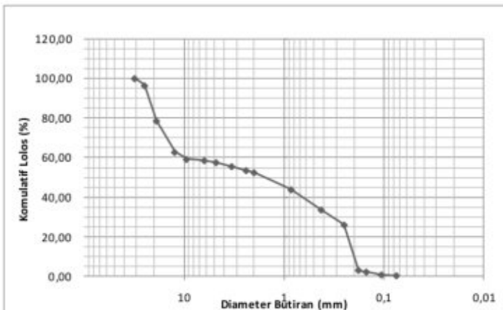
Gambar 9. Kurva Distribusi Kumulatif pada Pias 3 Survei II
