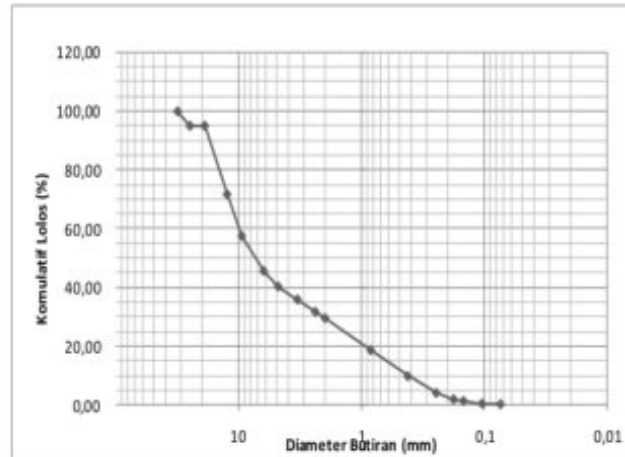
Gambar 6. Kurva Distribusi Komulatif pada Pias 3
