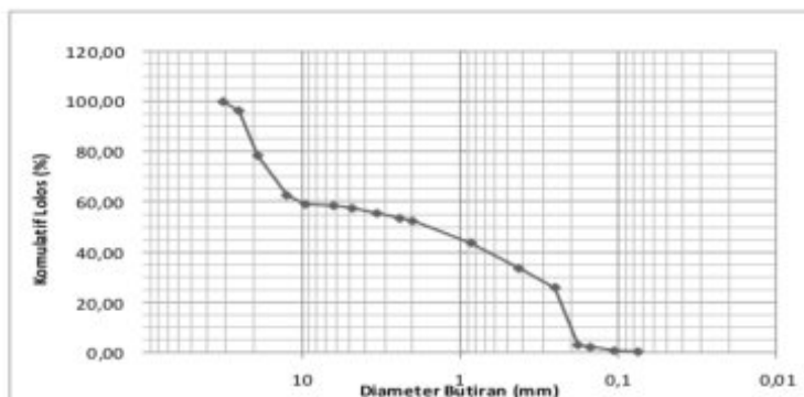
Gambar 7. Kurva Distribusi Kumulatif pada Pias 1 Survei II
