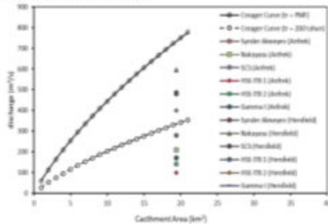
Gambar 6. Lengkung Creager DAS Bendungan Tanju
