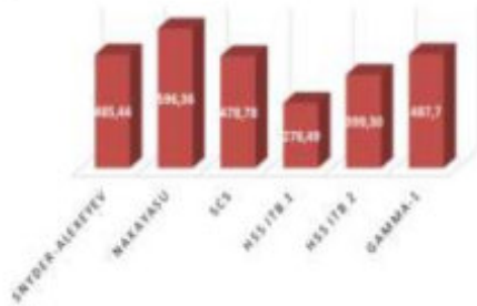
Gambar 5. Debit puncak PMF dari curah hujan PMP analisis frekuensi
