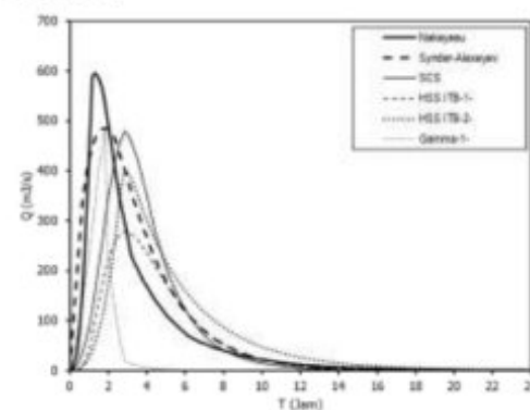
Gambar 4. HSS PMF dari curah hujan PMP Hersfield
