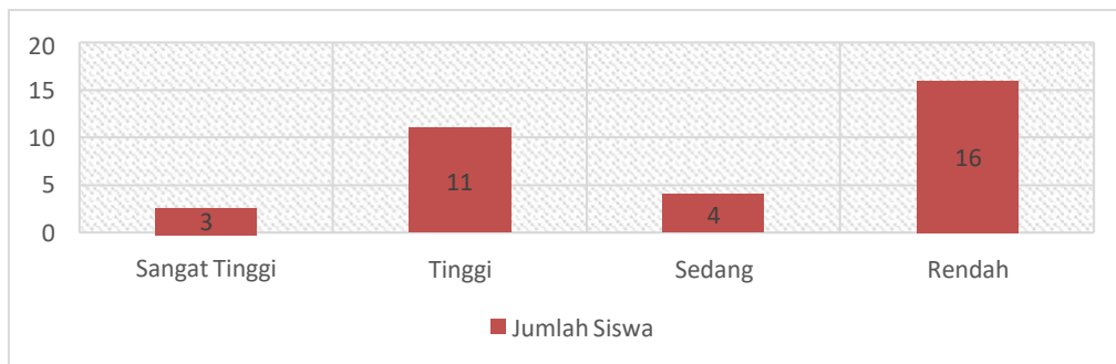
Gambar 1 Hasil Tes Rasio Trigonometri Siswa Kelas X MA Negeri di Lombok Timur Berdasarkan Kemampuan Awal Matematis Siswa
