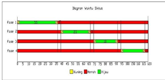
Gambar 4 Diagram Waktu Siklus Kondisi Eksisting Simpang Dasan Cermen
