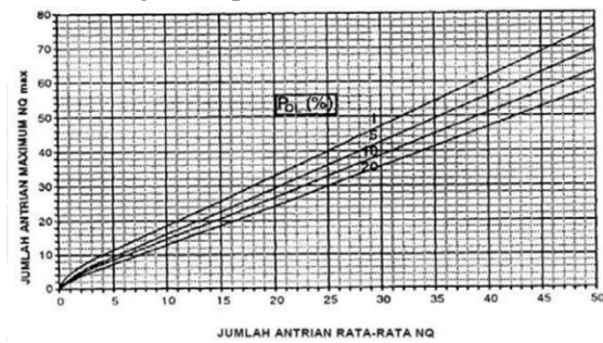
Gambar 1 Perhitungan Jumlah Antrian (NQ MAX ) Dalam smp
