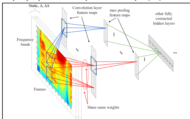
Gambar 2. Struktur CNN Untuk Pengenalan Suara
