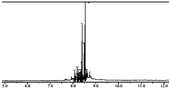
Gambar 3. Kromatogram GC Dengan Naungan
